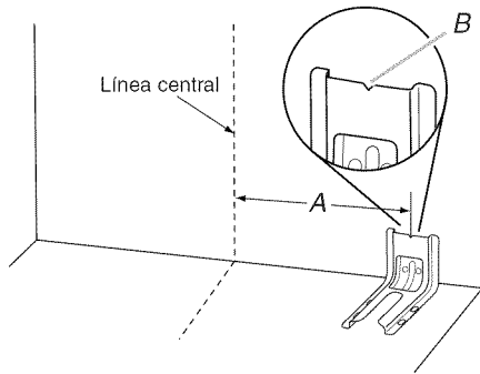
A. 12\frac{53}{64} " (32,6 cm) B. Muesca en V del soporte
