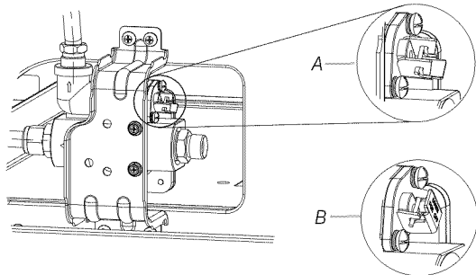
A. Posición de "Abierta" B. Posición de "Cerrada"
