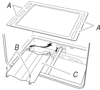
A. Bandeja del horno (levántela en el área mostrada para quitarla) B. Tornillos C. Esparcidor de llama
