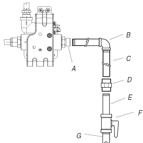
A. Accesorio de conexión del regulador de presión B. Codo de 90° C. Tubería de hierro negro
