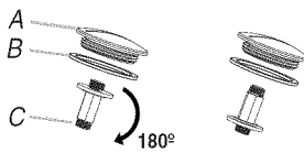
A. Tapa B. Arandela de sellado C. Tornillo de ajuste
