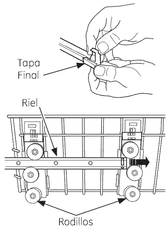
Estante Superior-Configuraciones de 10 lugares - GDF510 & GDF520
