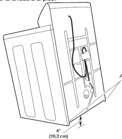
A. Patas autoajustables
