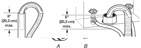
A. Acoplamiento B. Arandela
