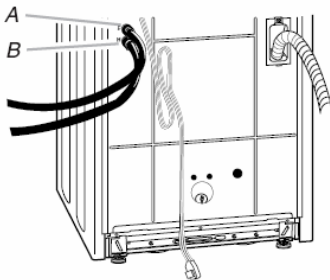
A. Válvula de entrada del agua fría (azul) B. Válvula de entrada del agua caliente (roja)
