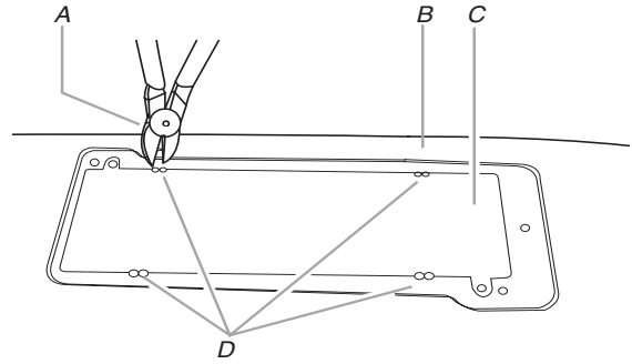
A. Pince coupante B. Sommet du four à micro-ondes C. Couvercle de fermeture de la bouche de sortie D. Points de fixation
