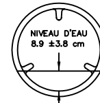
SANS CHARGE, POSITION DE DÉMARRAGE DU CYCLE POUR NIVEAU D'EAU 8.9 ±3.8 cm
