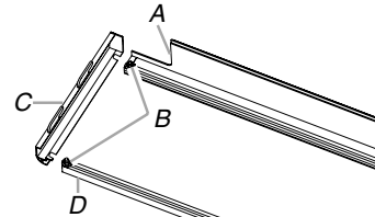
A. Riel inferior B. Tuercas C. Cubierta de borde D. Riel superior
