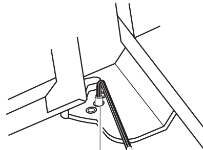
A. Vis de butée de porte
