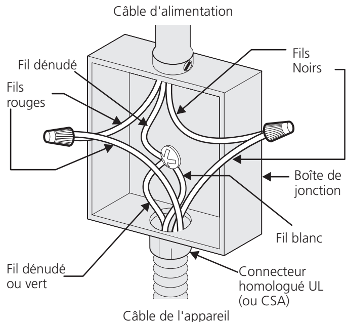
BOÎTE DE JONCTION À 3 FILS - MISE À LA TERRE Figure 6
