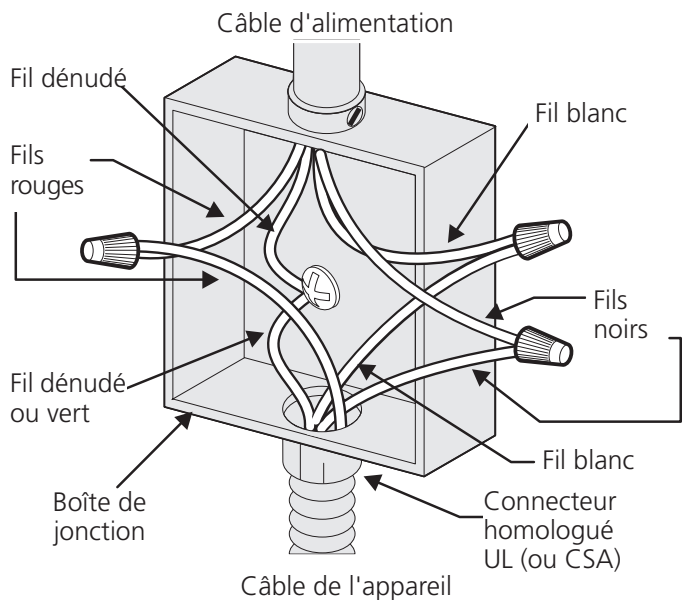
BOÎTE DE JONCTION À 4 FILS - MISE À LA TERRE Figure 7
