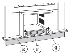
foam seal obturador de espuma joint de mousse cabinet gabinete caisse
