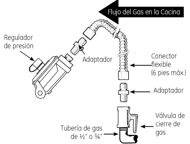
Tubería de gas desde la pared
