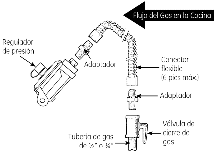
Tubería de gas desde el piso
