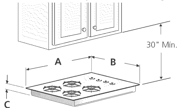
Dimensiones del hueco para la plancha de cocinar a gas
