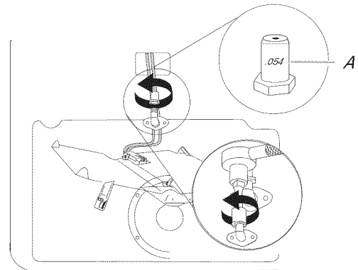
A. Injecteur femelle du brûleur de cuisson au grill pour gaz naturel - numéro 0.054
