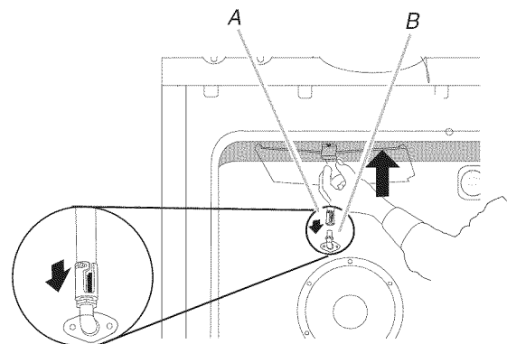
A. Injecteur femelle du brûleur de cuisson au grill B. Brûleur de cuisson au grill
