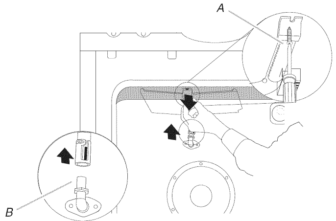
A. Vis du brûleur de cuisson au gril
