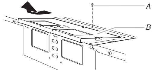
A. Tornillo B. Placa de la compuerta de tiro
