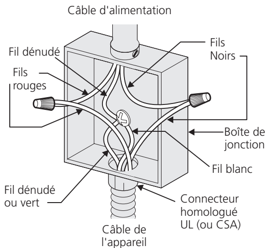
Figure 5 BOÎTE DE JONCTION À 3 FILS - MISE À LA TERRE
